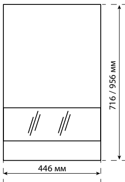
ВИТРИНА тип 1 (клееная)
