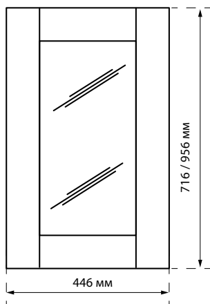
ВИТРИНА вертикальная (разборная)
